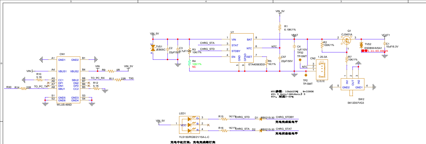
电源输入与电池充电
